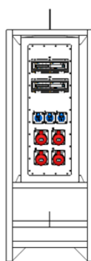
LATÉRAL
