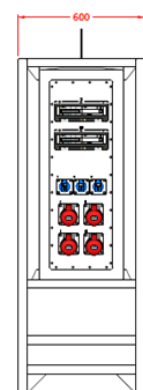
LATÉRAL
