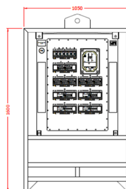
FACE
